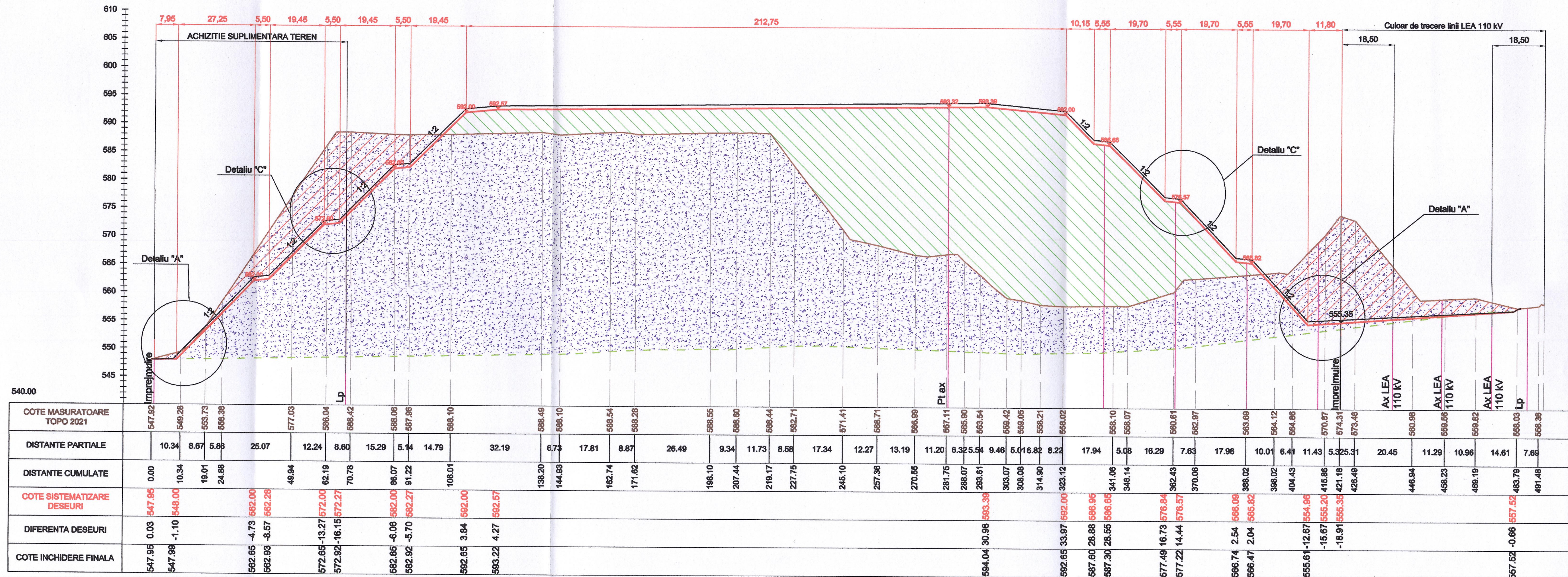
PROFIL LONGITUDINAL: Plax SCARA: 1:1000/1:500
